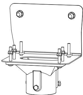
Stolpfäste 353687/353688
